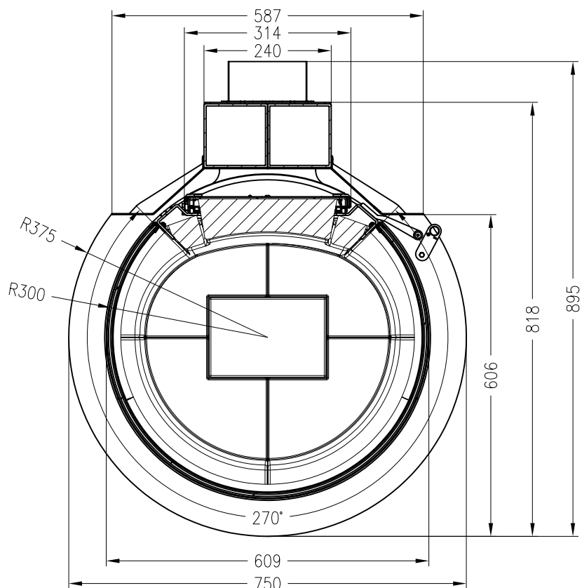
Horizontalschnitt M ~1:10
