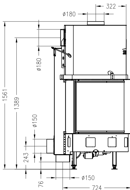
Seitenansicht M ~1:20
